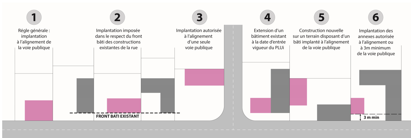
Schémas illustratifs d'implantations possibles des constructions vis-à-vis des voies et emprises publiques, Réalisation APGL
